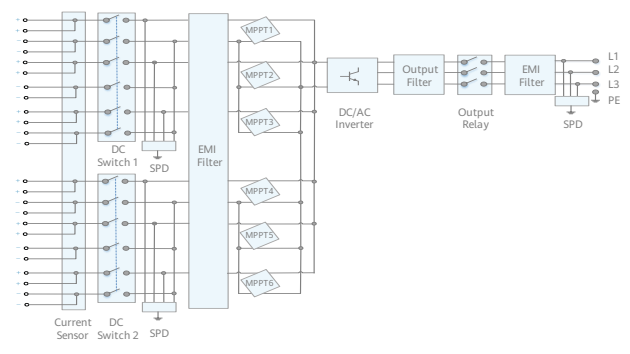
SUN2000-50KTL-M0
